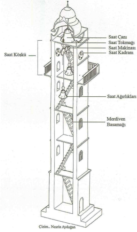
Çizim.. Nesrin Aydoğan Çiz.2, Kule Saatinin Bölümleri, Hakkı Acun'dan
