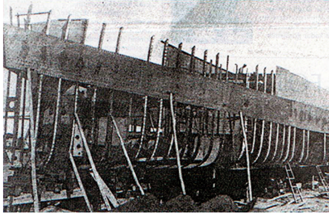
Resim 6: Geminin Sac Havuza Alınması
