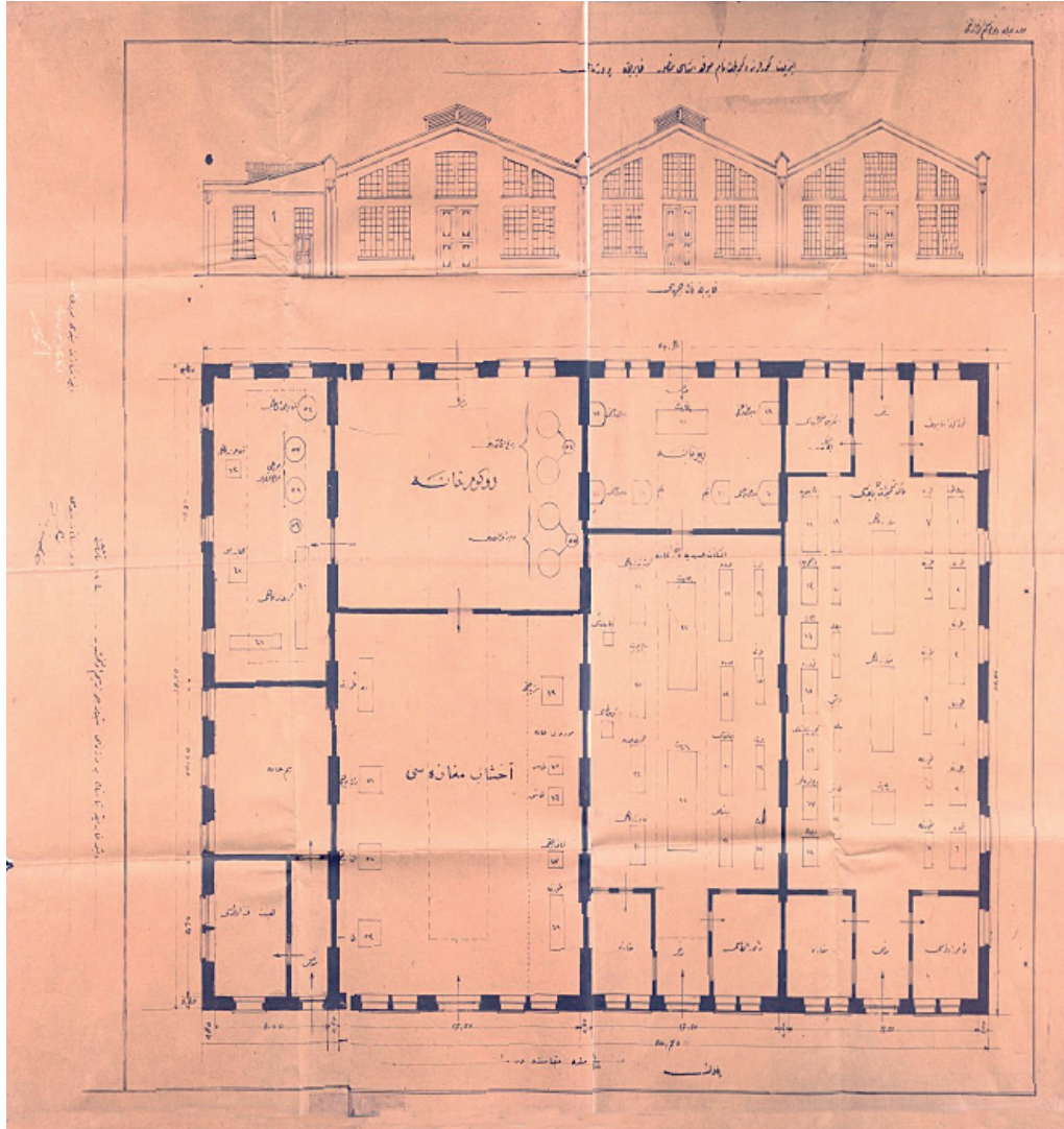
Resim 4: Tersane Planı 56
