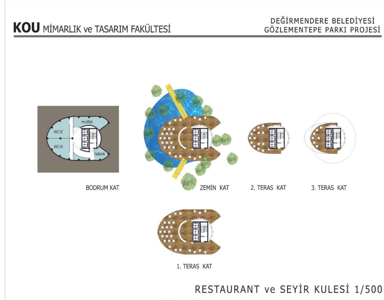
Şekil 3. Kat Planları
