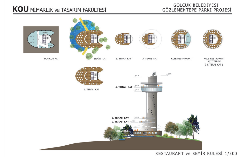
Şekil 2. Kat Planları ve Kesit
