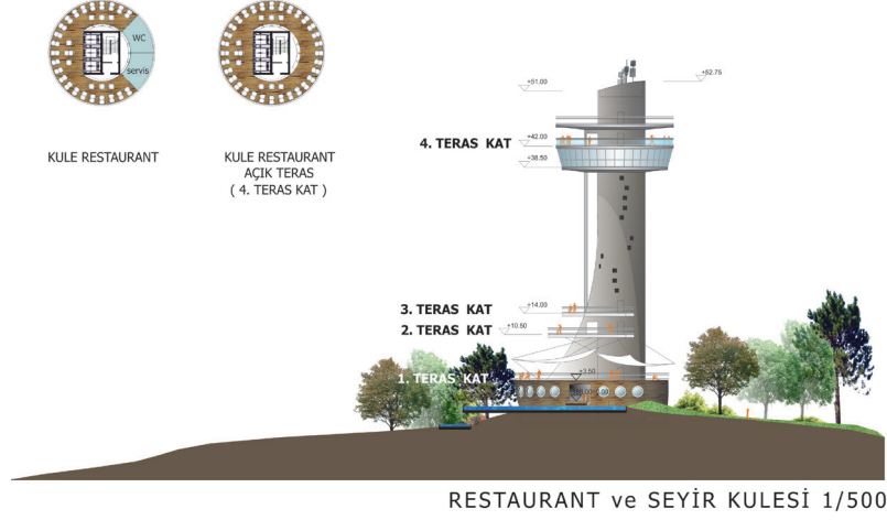
Şekil 4.Kesit
