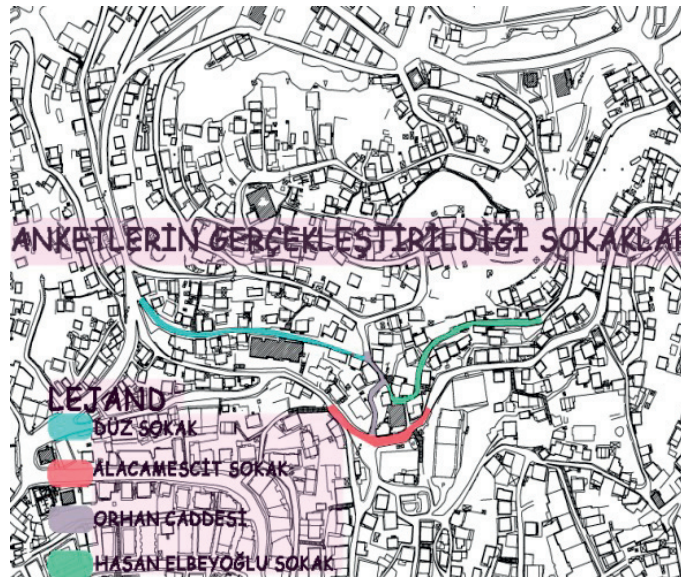
Şekil 2. Akçakoca mahallesi yerleşimi ve sokaklarının kısmi vaziyet planı
